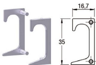
PUNTERA ALT 10 (PAR) LAT IZQ/DER ANODIZADO 15 mm
