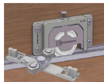
KIT PUERTA ALT - AL 52 CUERPO NAILON RODILLO SUPERIOR AUTOAJUSTABLE GA06
