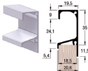
PERFIL JALADOR ALT 5047T
