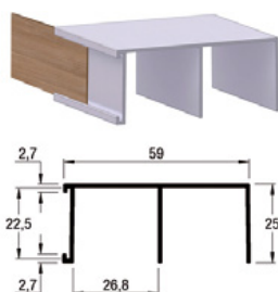
RIEL SUPERIOR ALT 3055 ANODIZADO TAPACANTO
