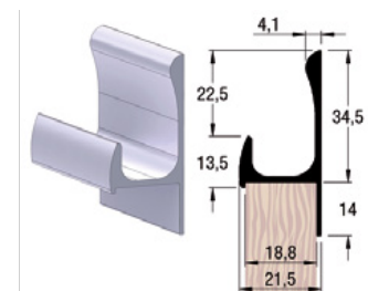
PERFIL JALADOR ALT 5017 ANODIZADO P/ TABLERO 18 mm
