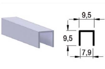
PERFIL ALT 2080 TAPACANTO U 7.9 mm
