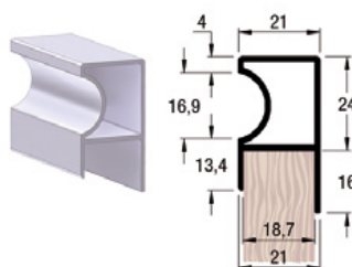
PERFIL JALADOR ALT 4004 ANODIZADO PERFIL JALADOR ALT 4002 ANODIZADO
