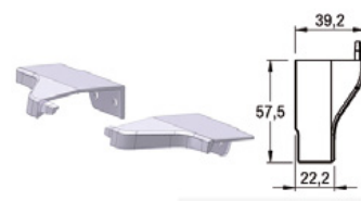
PUNTERA ALT 12 (PAR) LAT IZ/DER AREZZO INOX ESCOBADO 18 mm
