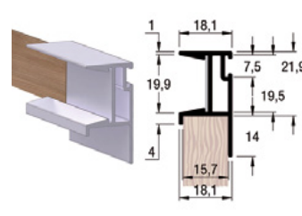
PERFIL JALADOR ALT 4101 ANODIZADO TAP. PERFIL JALADOR ALT 4102 JAT ANOD P/TABL.
