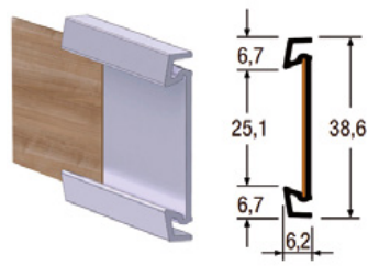
PERFIL JALADOR ALT STRETTO ADHESIVO
