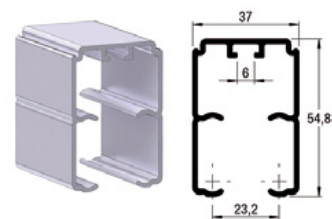
PERFIL SUP ALT 2083 ANODIZADO
