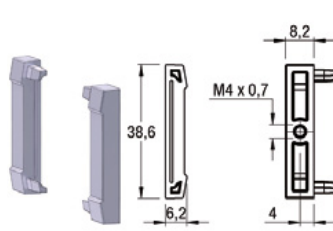
PUNTERA ALT 19 (PAR) LAT IZQ/DER STRETTO ANODIZADO 18 mm
