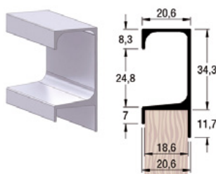
PERFIL JALADOR ALT 5047 ANODIZADO PERFIL JALADOR ALT 5046 ANODIZADO
