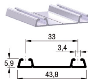
RIEL INFERIOR ALT 1052 ANODIZADO
