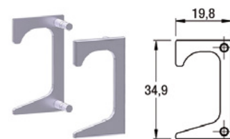
PUNTERAS ALT 07 DER/IZ PARA PERFIL 5047T
