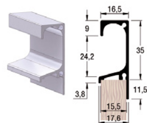
PERFIL JALADOR ALT 4016T ANOD P/ TABL 15 mm
