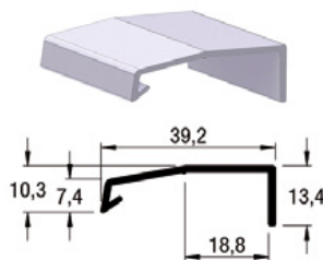
PERFIL JALADOR ALT AREZZO INOX ESCOVADO 18 mm
