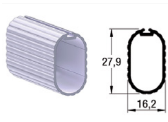
TUBO COLGADOR OVALADO ALT
